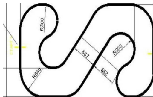
Чертёж поля для проекта «Траектория»
